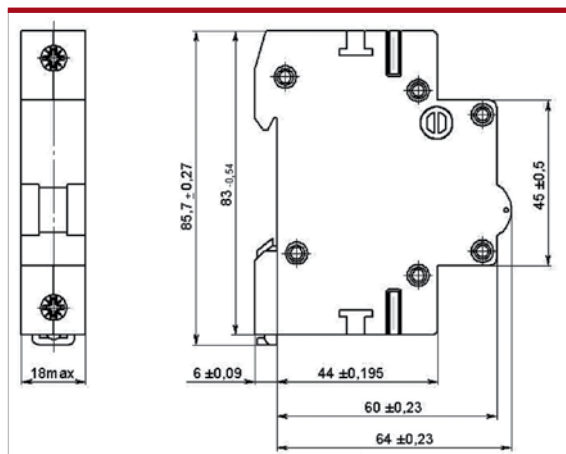
Габаритные размеры OptiDin ZM63
