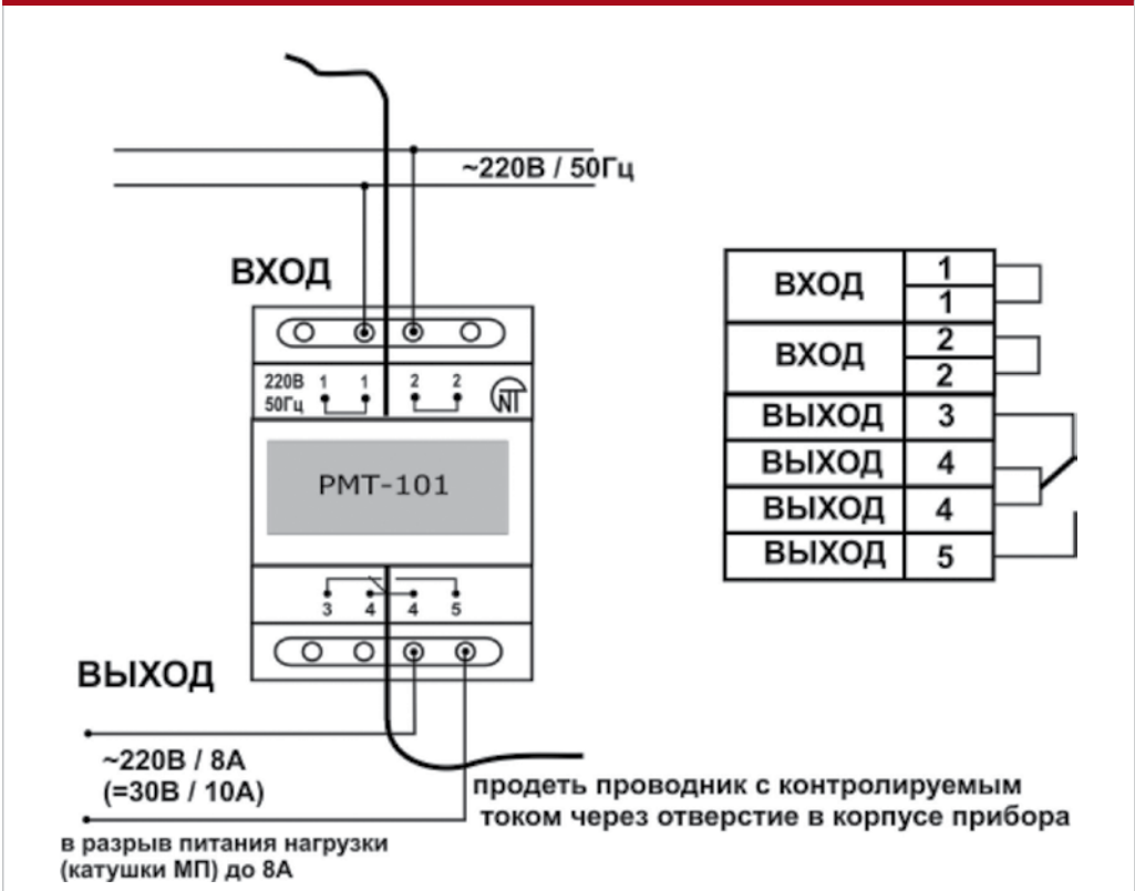
Схема подключения реле OptiDin PMT-101
