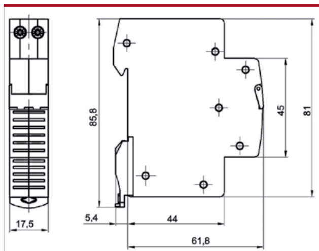
Габаритные размеры OptiDin ZM63
