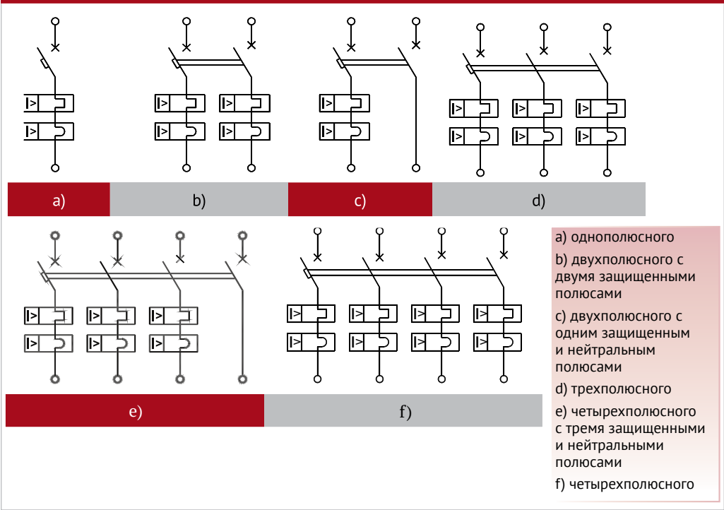
Принципиальные электрические схемы автоматических выключателей OptiDin BM63
