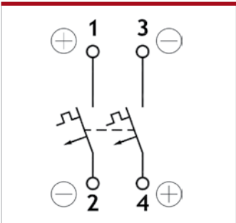
2-полюсный OptiDin BM63 DC
