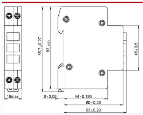
Габаритные размеры OptiDin SL63
