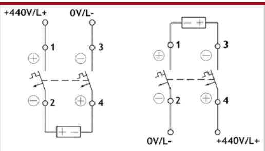
2-полюсный OptiDin BM63 DC
