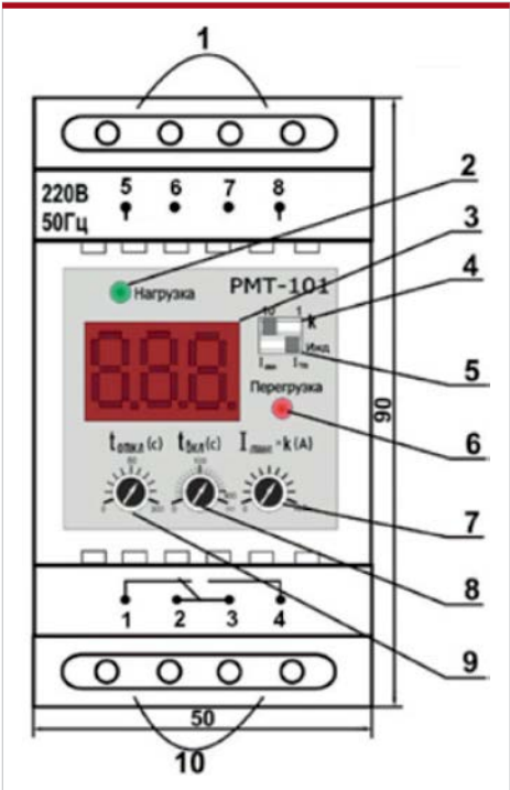
Схема подключения реле OptiDin PMT-101
