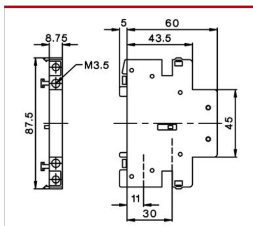
Блок вспомогательных контактов OptiDin RH11
