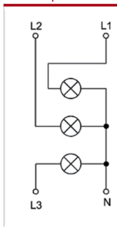
Принципиальная электрическая схема OptiDin SL63
