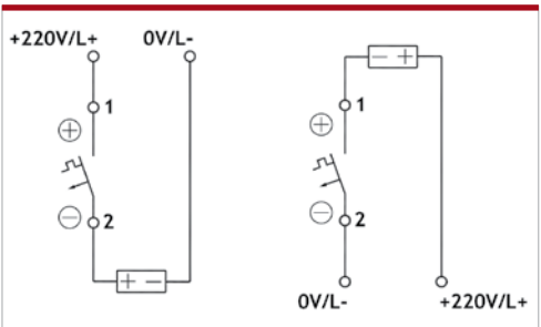
1-полюсный OptiDin BM63 DC
