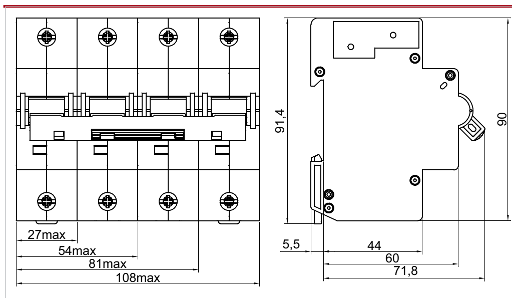
Габаритные, установочные и присоединительные размеры автоматических выключателей OptiDin BM125
